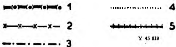
Fig. 1. Usytuowanie powiatu ustrzyckiego w dawniejszym podziale administracyjnym, 1 : 500 000. 1 — granica państwa, 2 — granica państwa w latach 1944—1951, 3 — granica powiatu, 4 — granice powiatów w r. 1931, 5 — linia kolejowa
